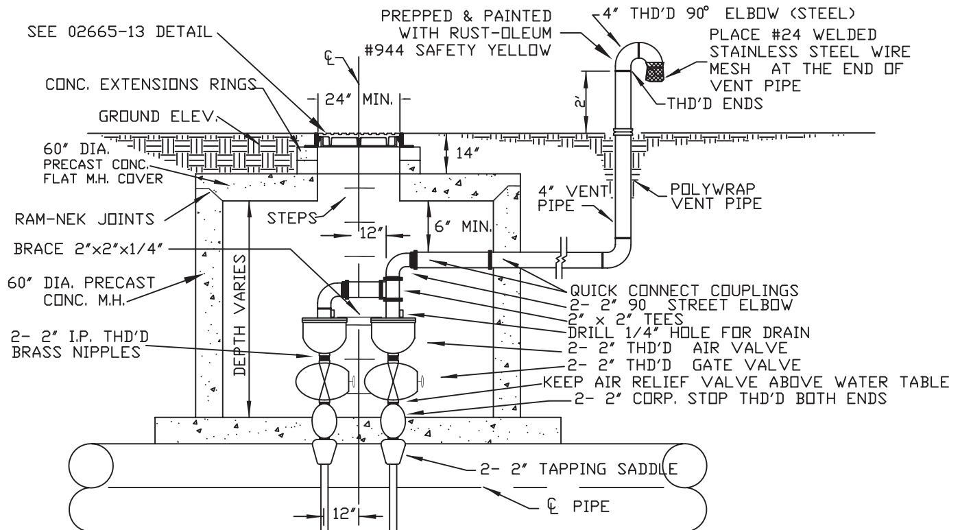
ELEVATION
