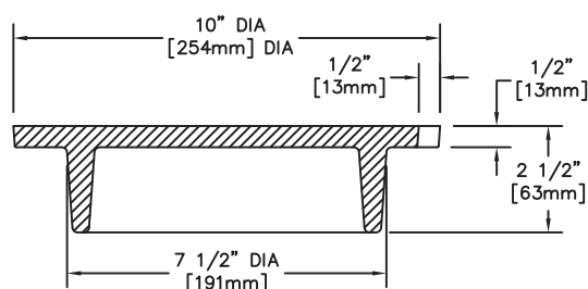
LID DETAIL
